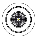
luminária: Ø 140 mm nicho: Ø125 mm
